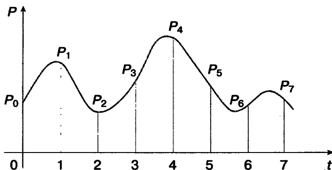
Рис. 1.9. Барограмма
